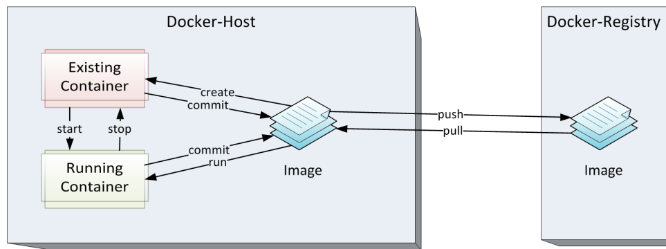
Abbildung 1: Docker-Lebenszyklus (vereinfacht)
